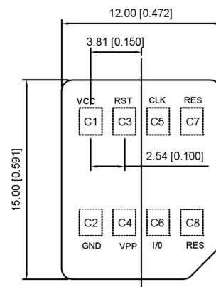
MICRO SIM CARD 芯片面朝下视图
