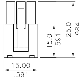
3 CIRCUITS
