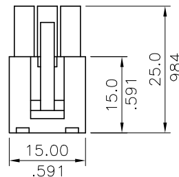
6 CIRCUITS
