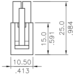
2 CIRCUITS
