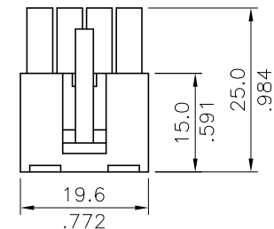
12 CIRCUITS
