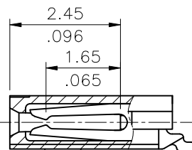
SEC.:Y-Y
