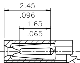
SEC.:Y-Y
