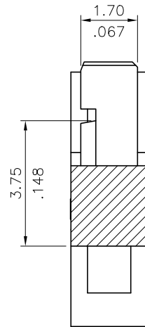
SEC. A-A
