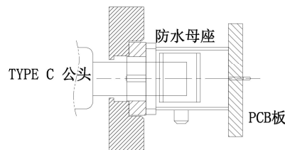
组装示意图
