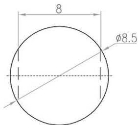
取付穴参考寸法 Mounting hole dimension
