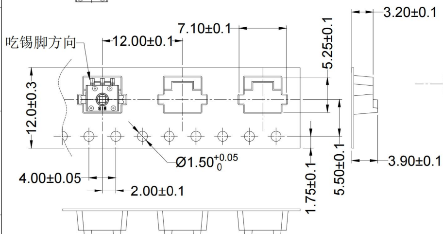
图2 成品载带
