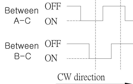
(SW01) OUTPUT
