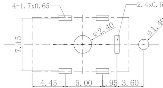
PCB板开孔尺寸
