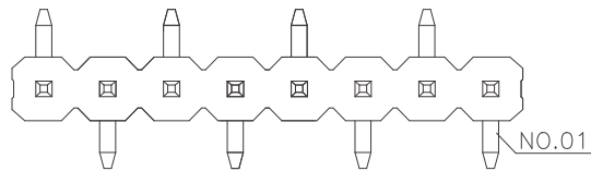
R1 TYPE
