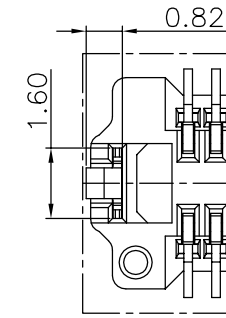
DETAIL B 2:1
