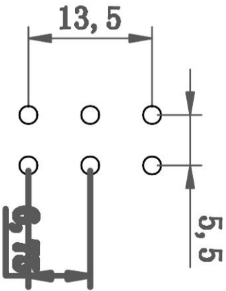
开孔尺寸
