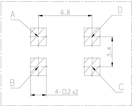
焊盘尺寸
