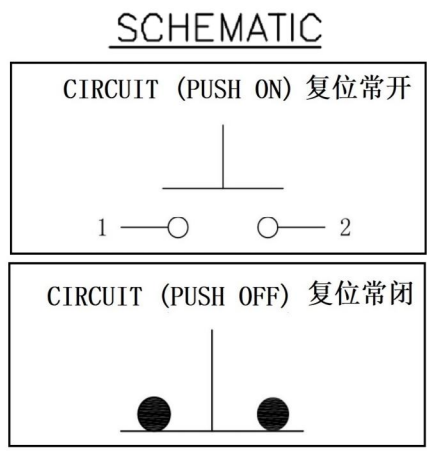
电气原理图
