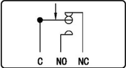
电器原理图
