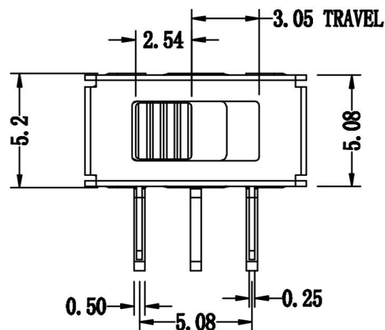
ACTUATOR IN POS. 1
