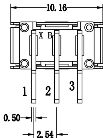
ACTUATOR IN POS. 1
