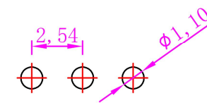
安装孔尺寸
