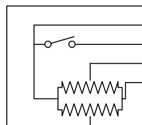
接线图 Circuit Explanation
