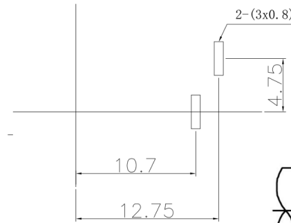
线路板安装尺寸示意图
