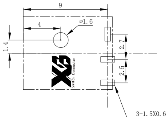
线路板开孔尺寸
