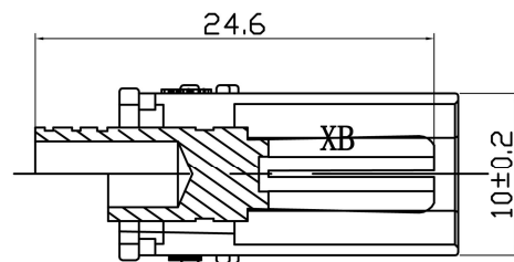
截面 A-A
