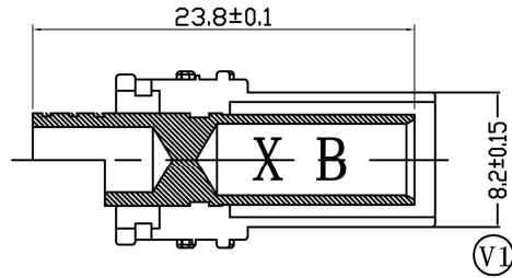
截面 A-A
