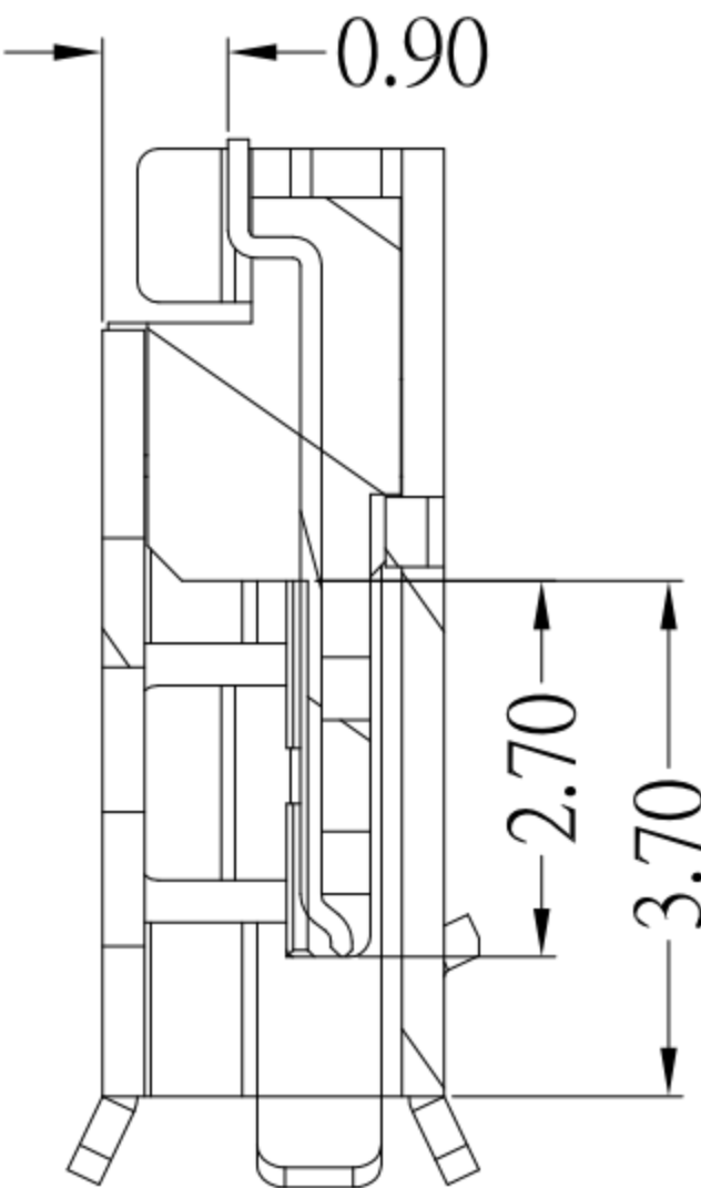
剖面 A-A
