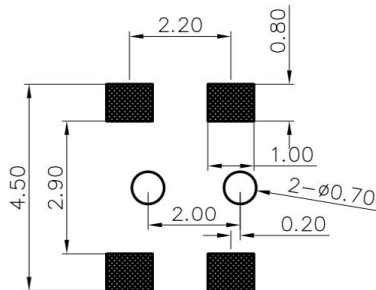
安装尺寸
