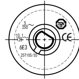
外壳字唛图
