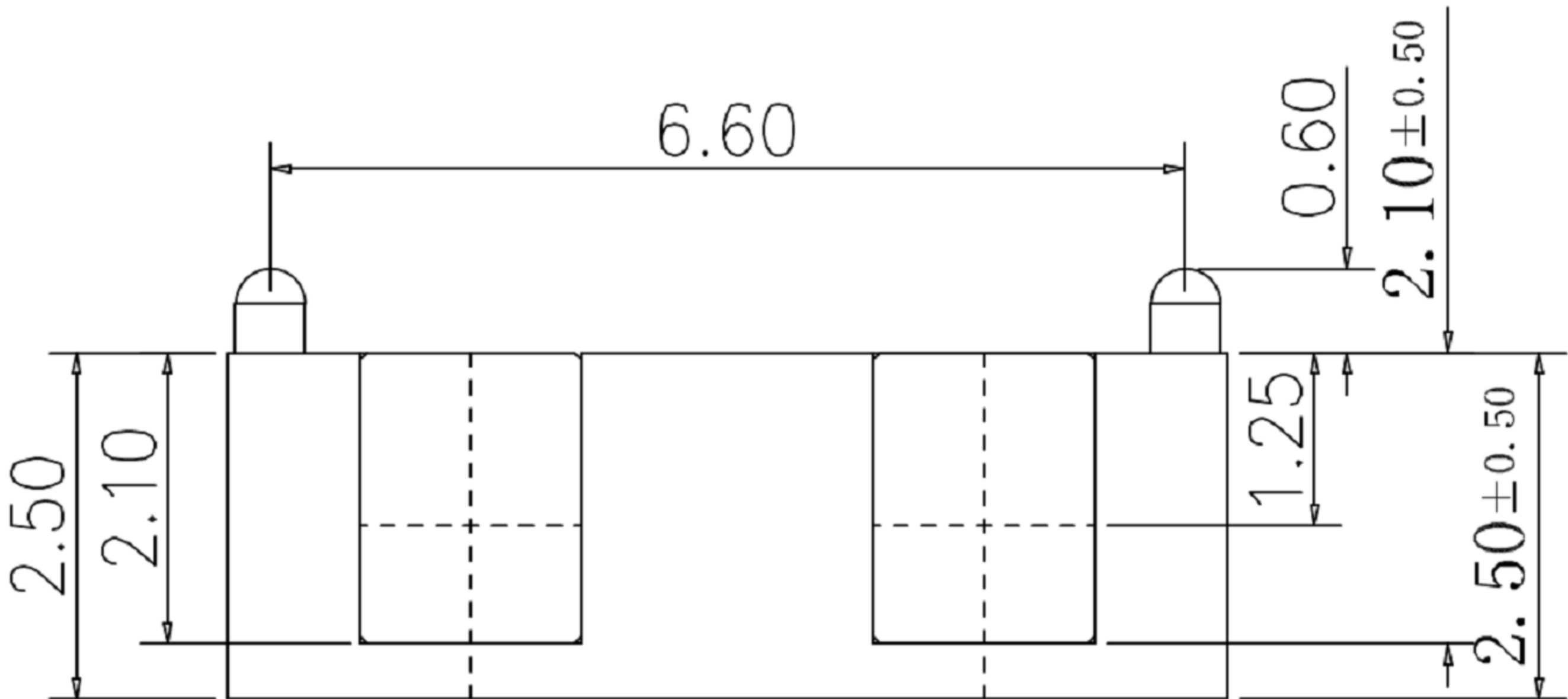
图为焊盘位置和大小
