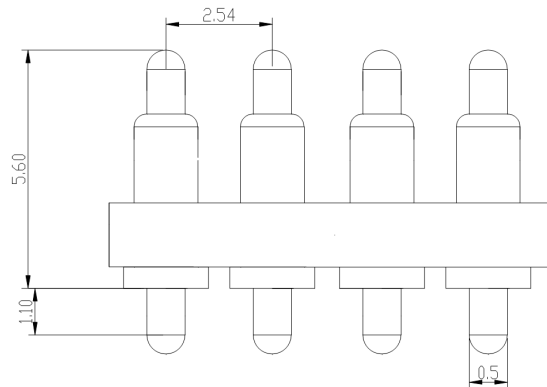
图为焊盘位置和大小
