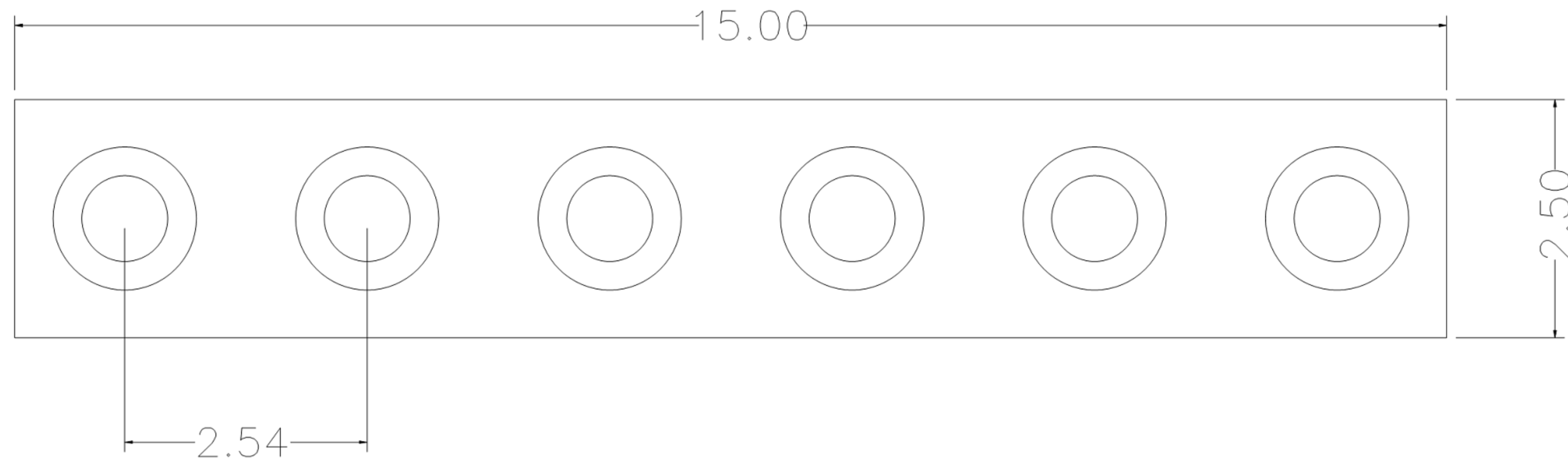
图为焊盘位置和大小
