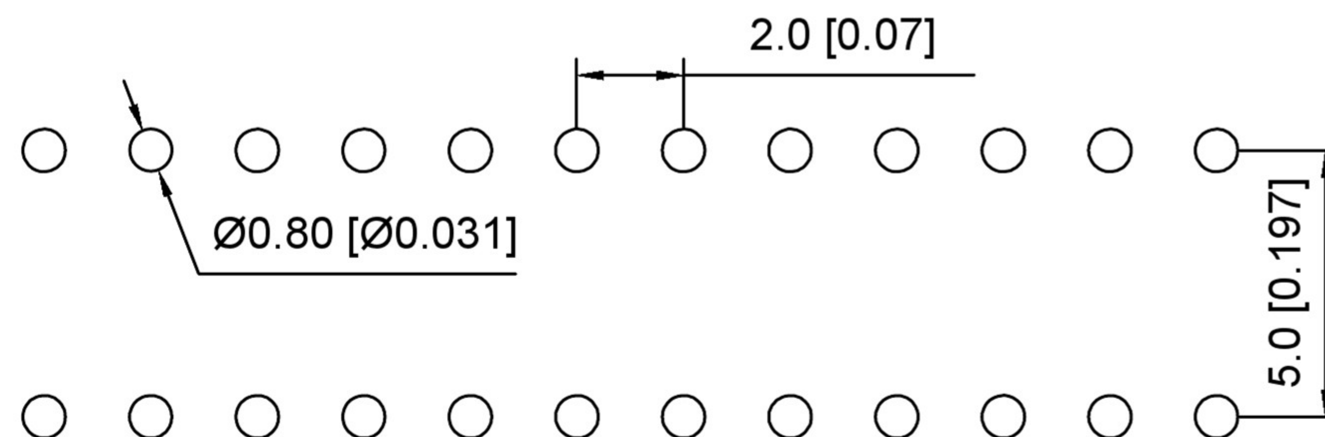
P.C.B LAYOUT
