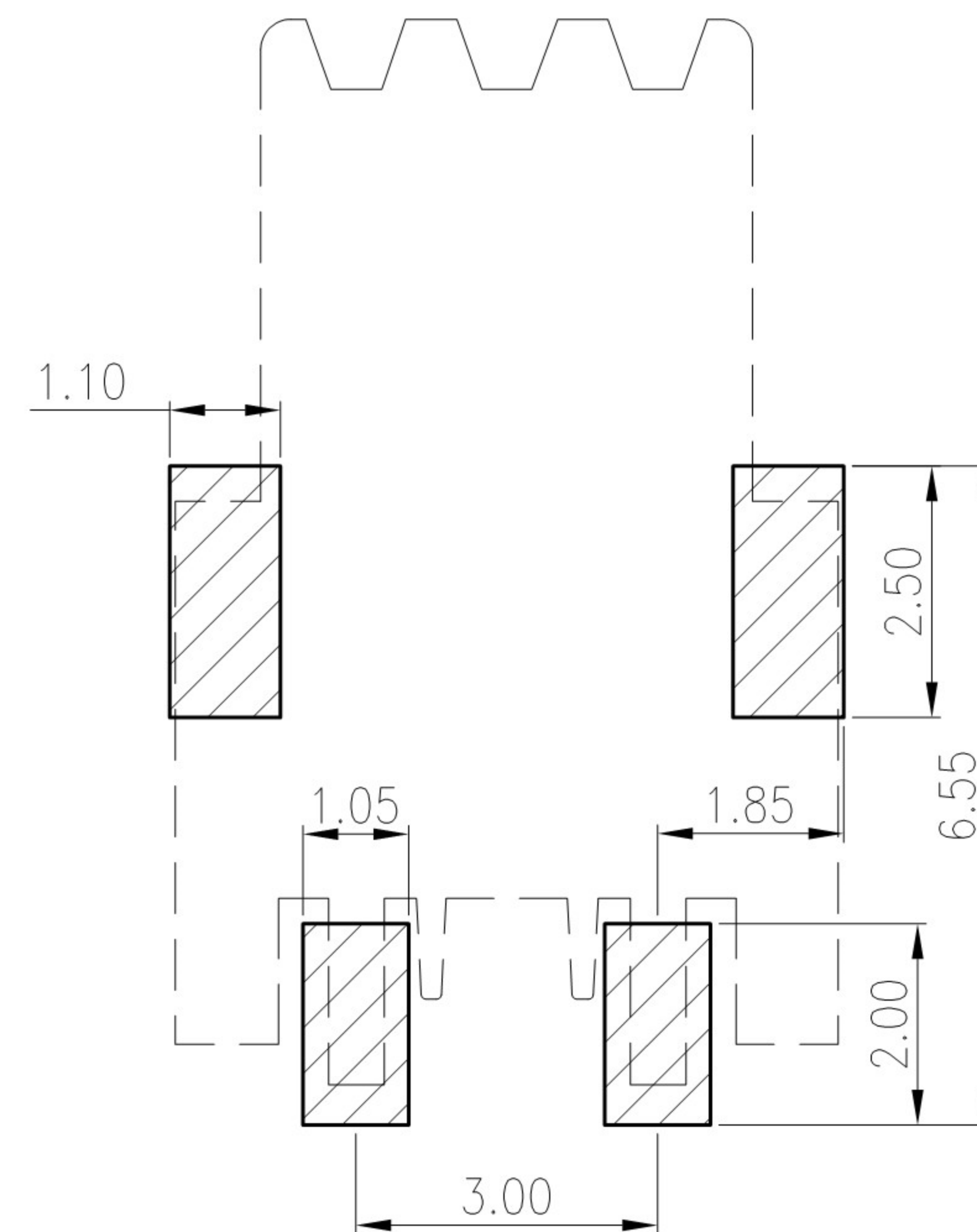
P.C.B Layout
