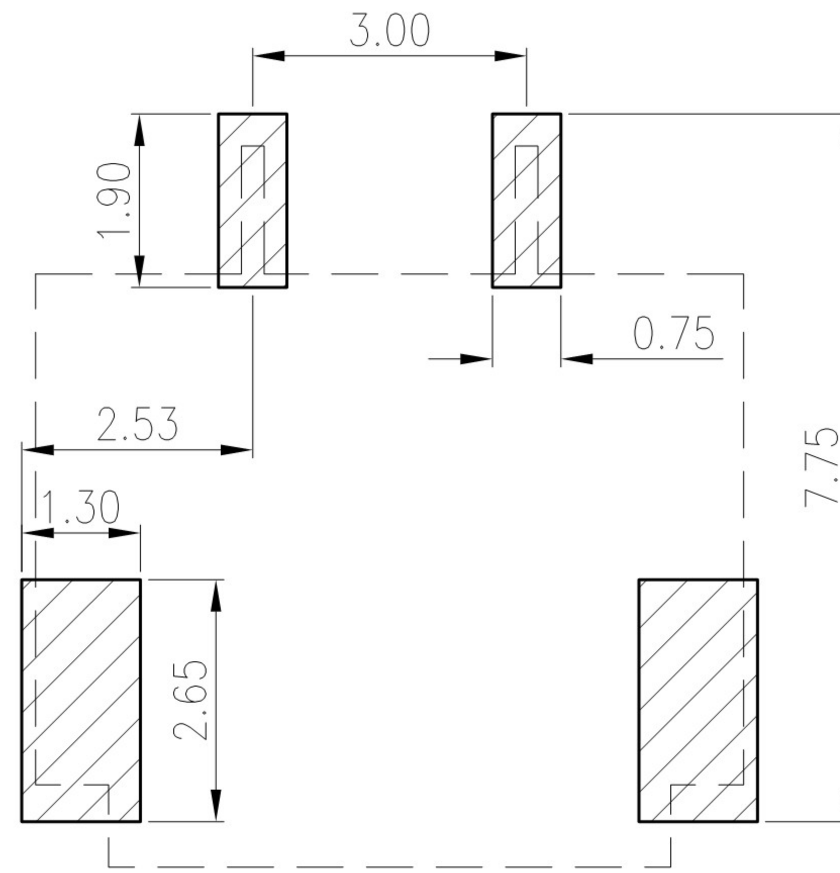
P.C.B Layout
