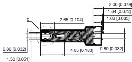
SECT A-A
