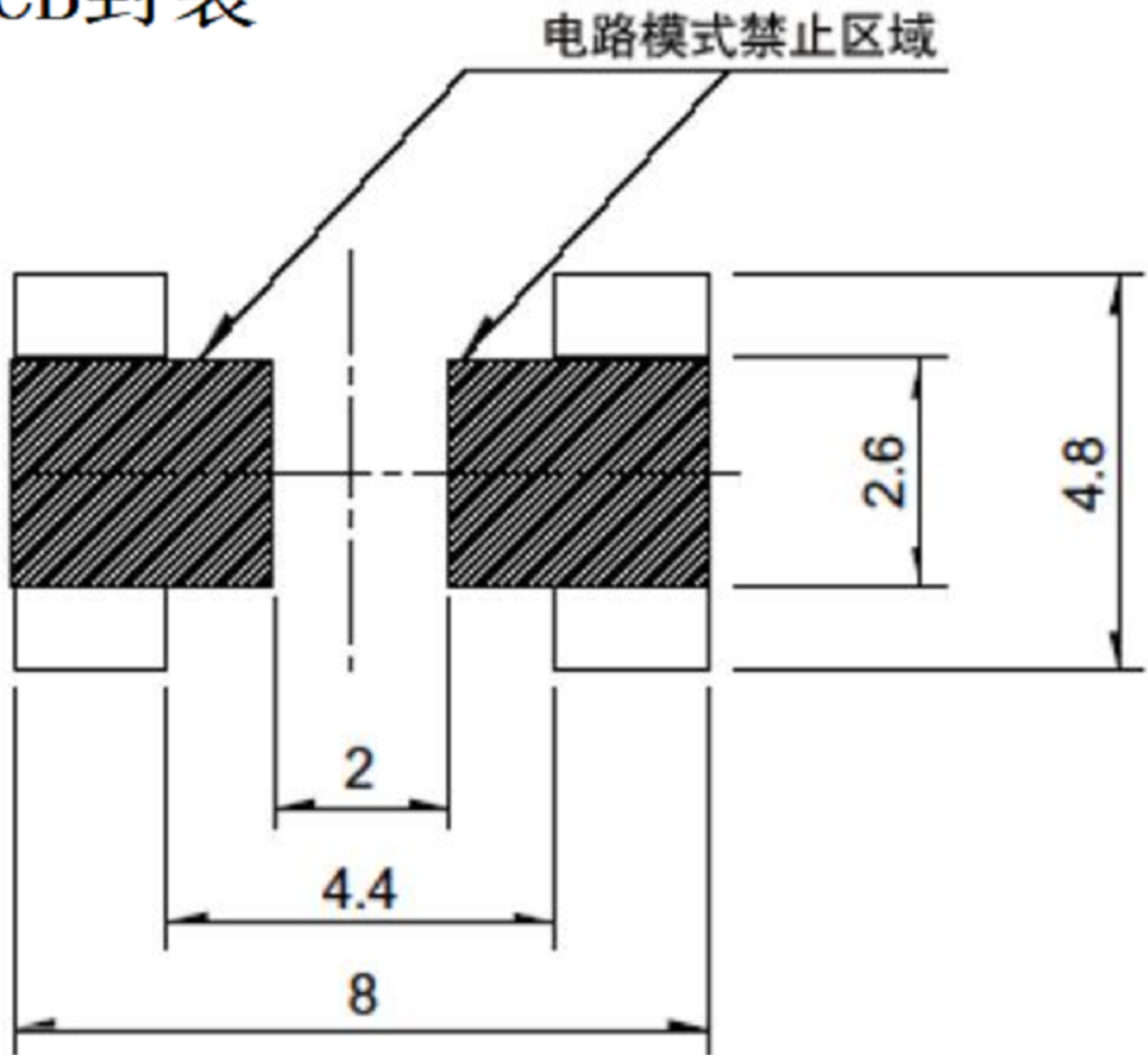
PCB封装
