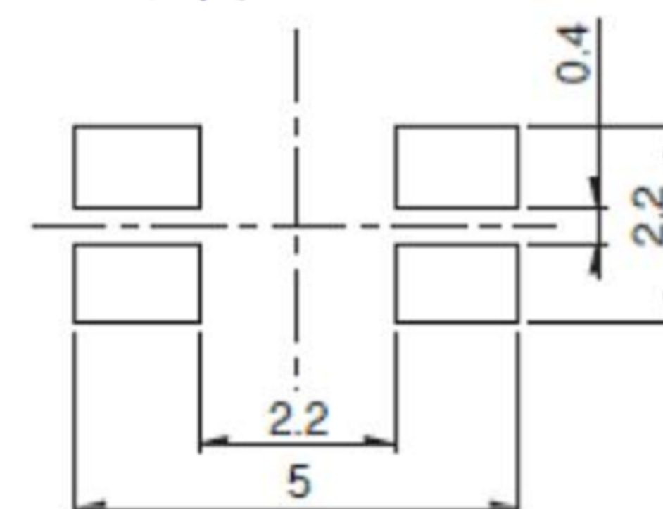
PCB封装
