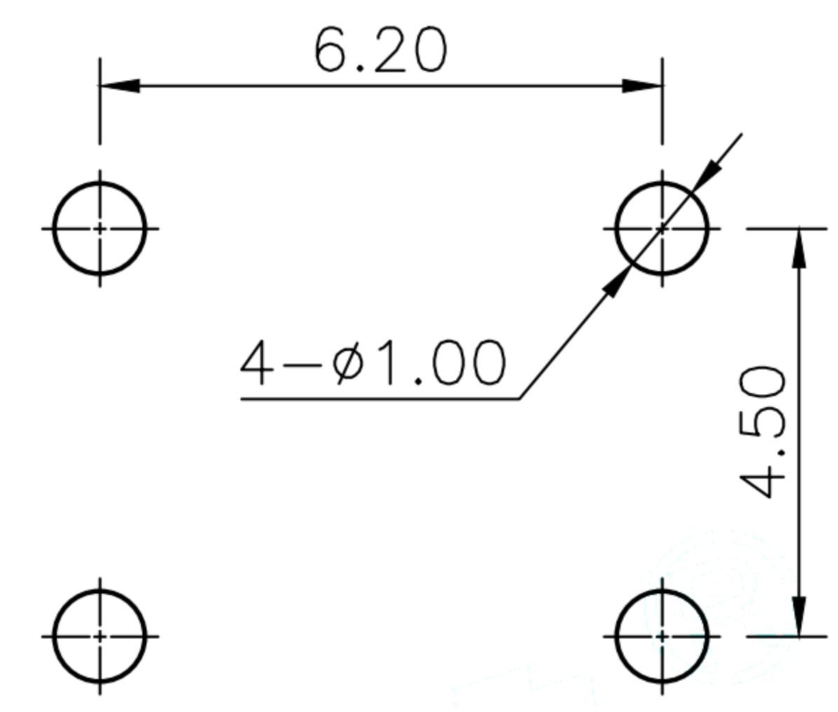
PCB Layout(Pattern side)
