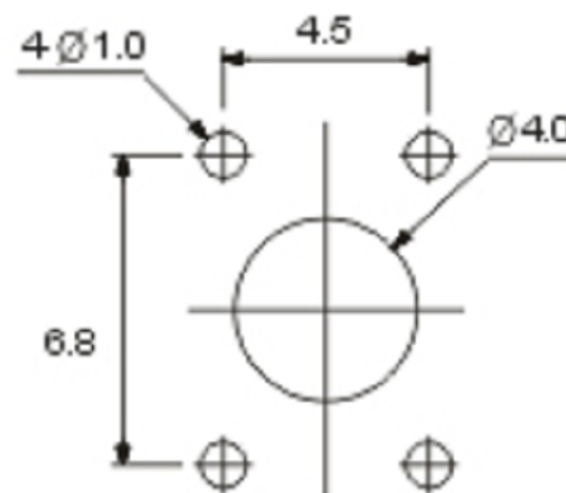
P.C.B HOLE DIMENSION
