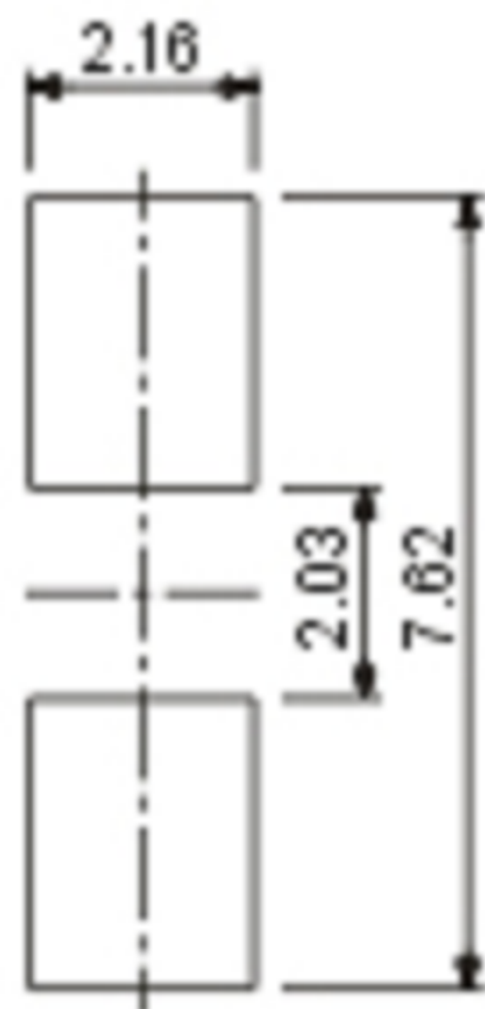
P.C.B LAND DIMENSION
