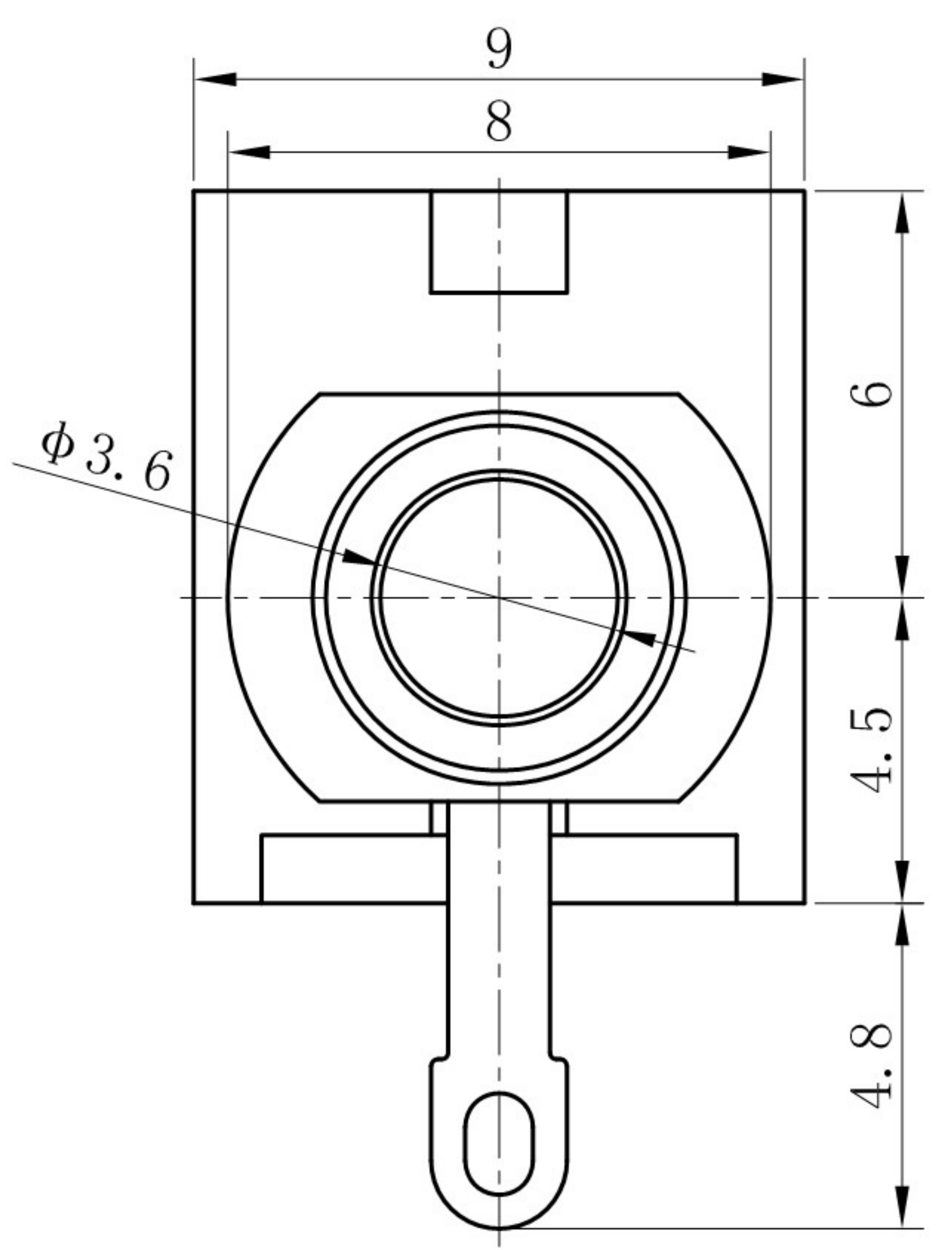
线路板开孔尺寸 P.C.B LAYOUT
