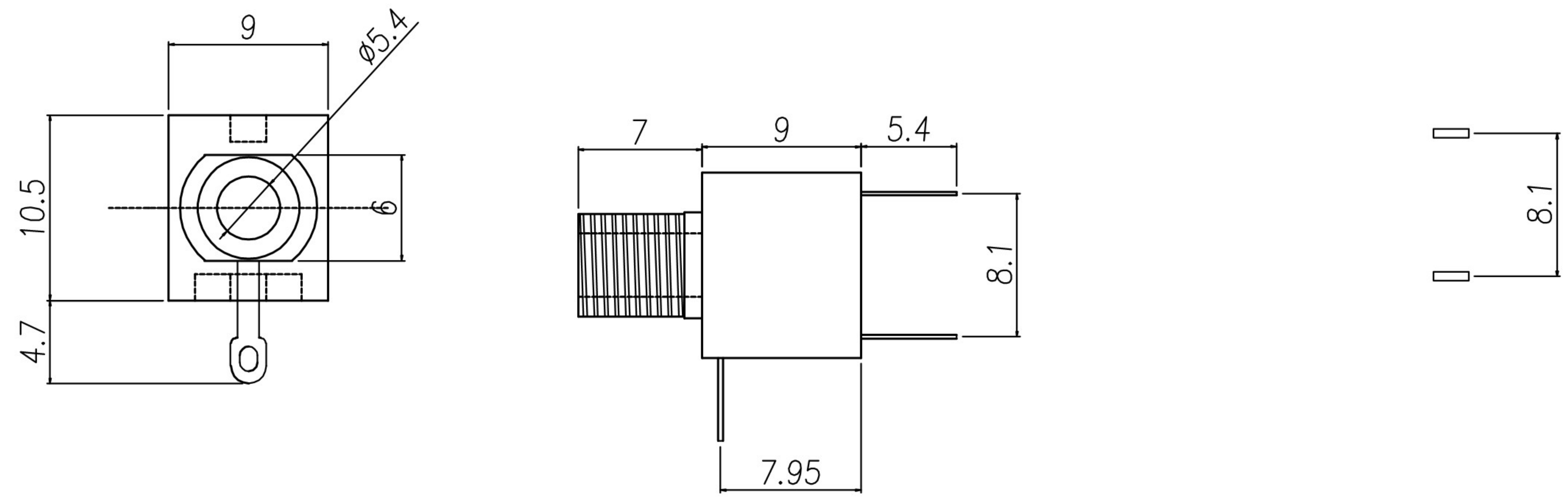
线路板安装尺寸示意图
