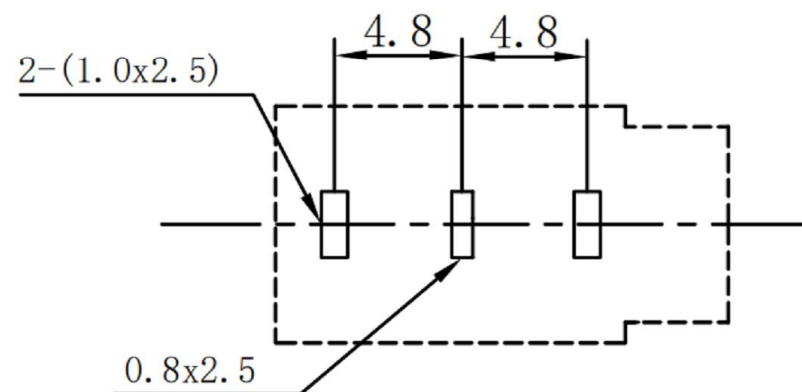
线路板安装尺寸
