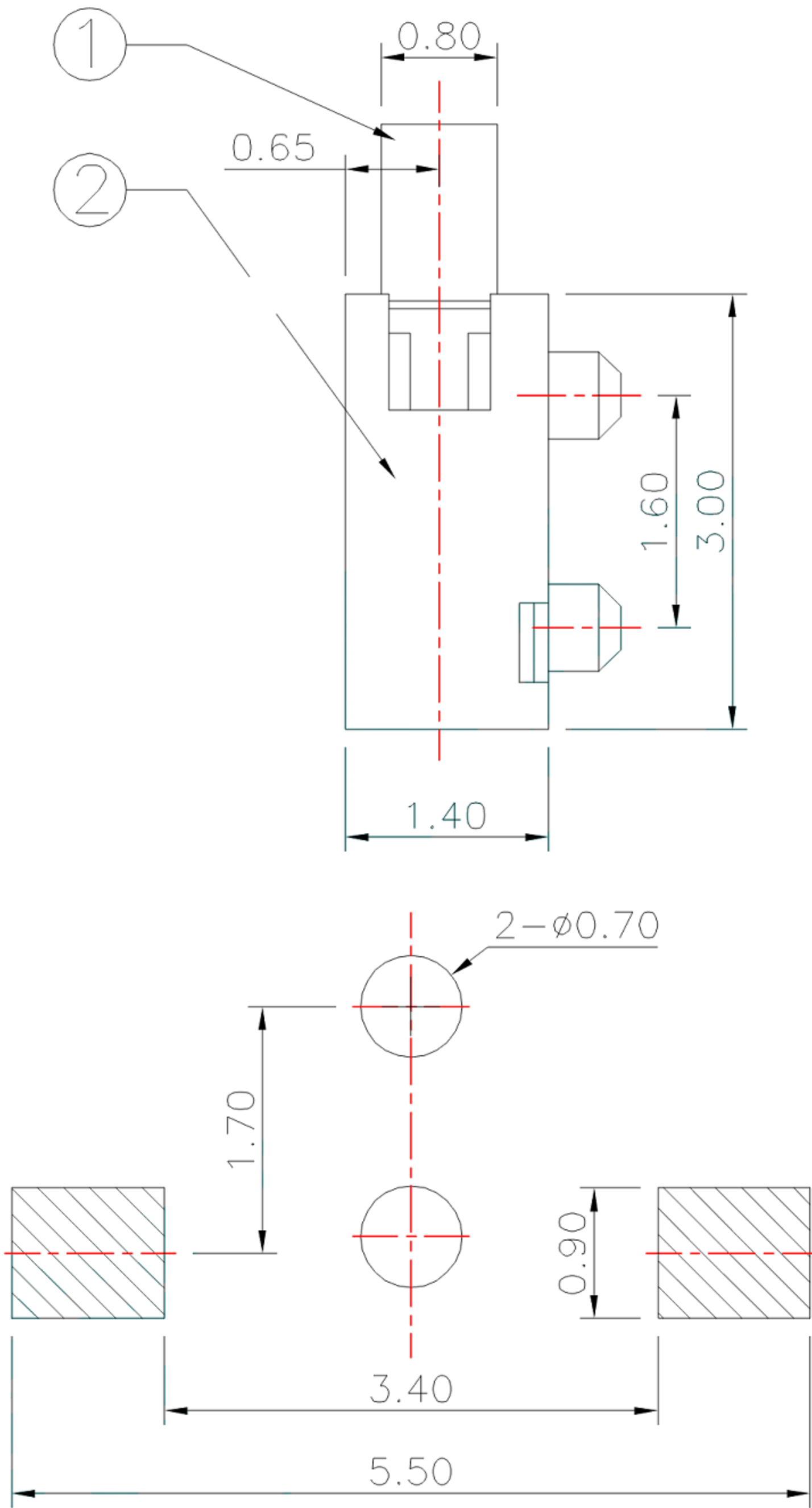
PCB Layout(Pattern side)
