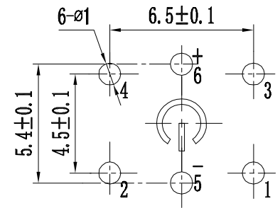
元件面孔位图
