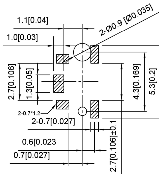
P.C.B LAYOUT
