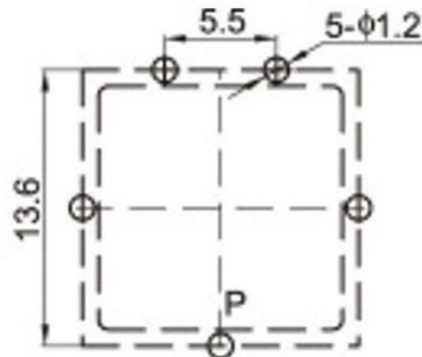
印制线路板 P.C.B
