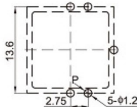
印制线路板 P.C.B
