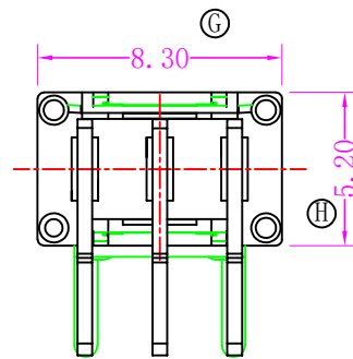
手柄位置及导通端子示意图
