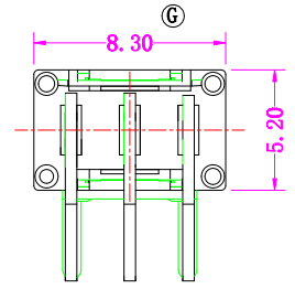
手柄位置及导通端子示意图
