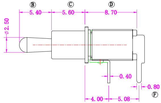
标注：(A) - (G) 尺寸的重点检验尺寸
