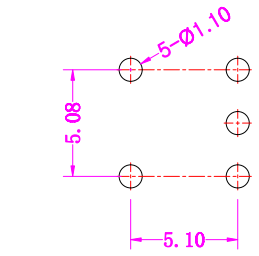
安装孔尺寸
