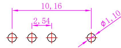
安装孔尺寸
