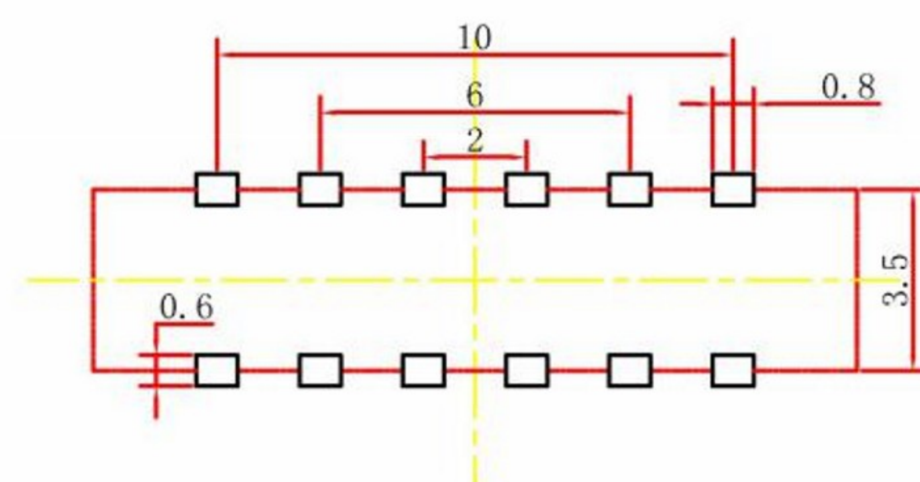
PCB板位置尺寸
