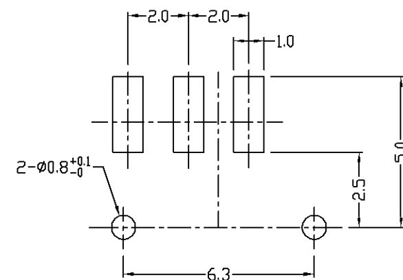
P.C.B. LAYOUT
